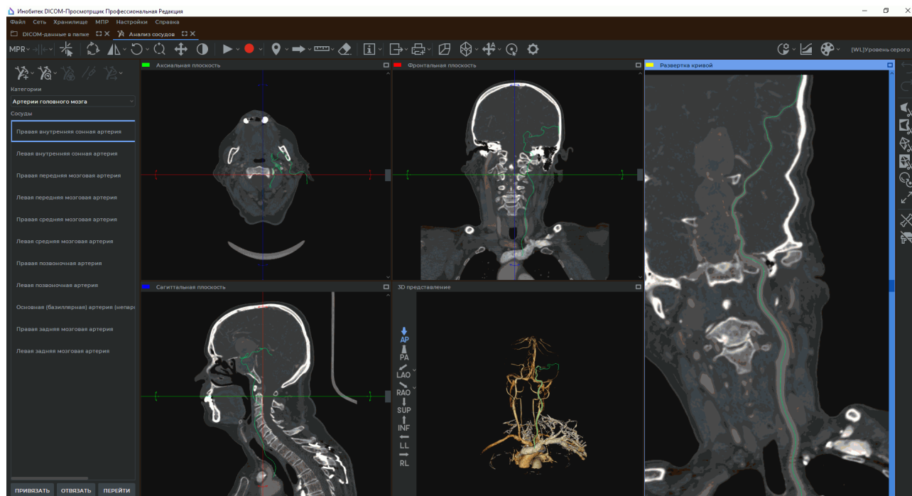
Рис. 7.5: Центральная линия
