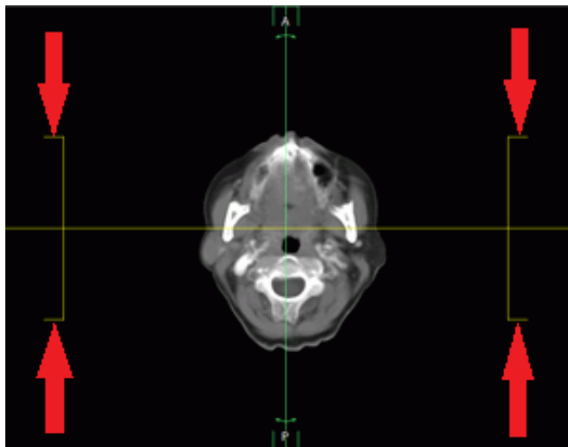
Рис. 5.24: Границы слоя
