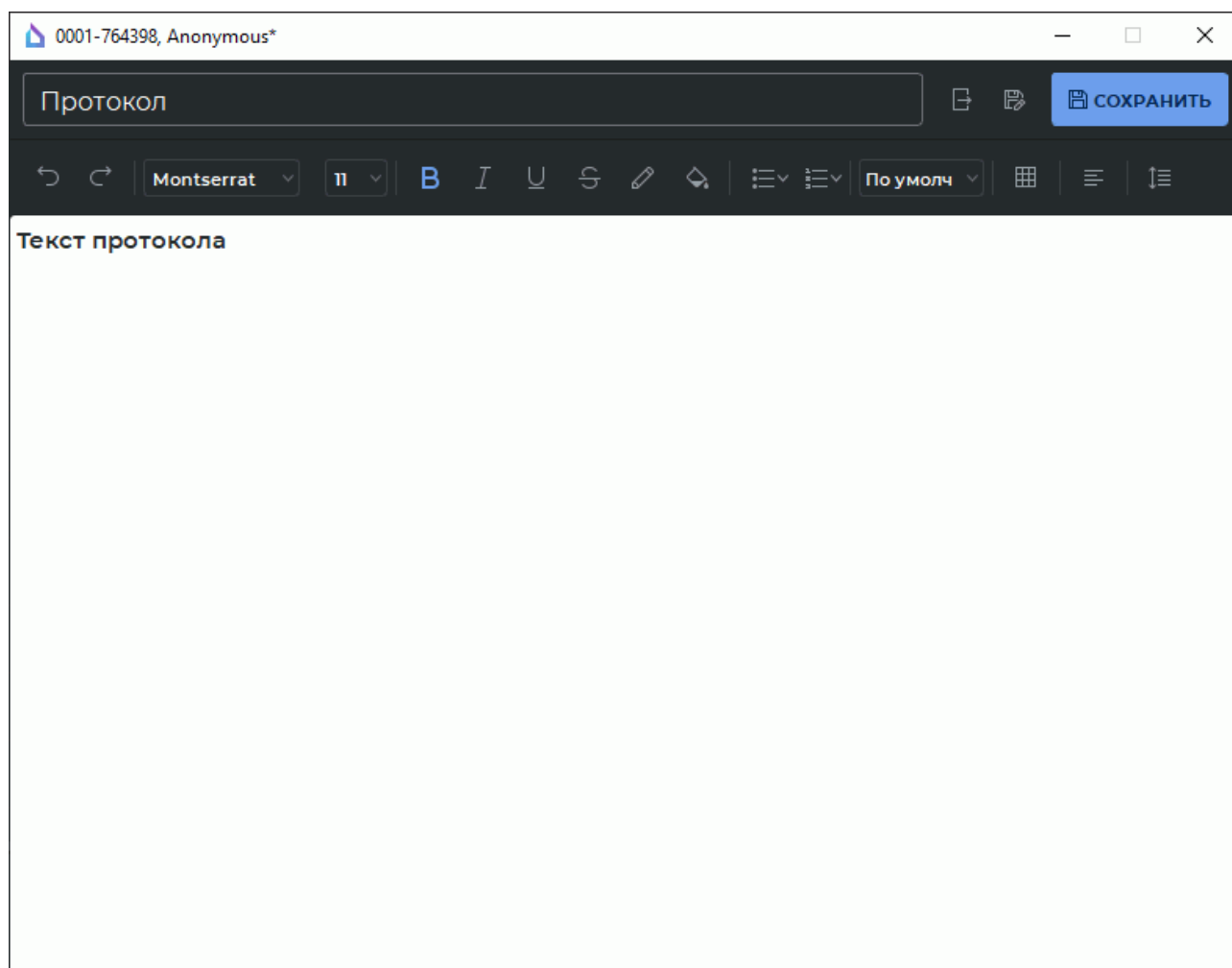
Рис. 18.1: Окно редактора
