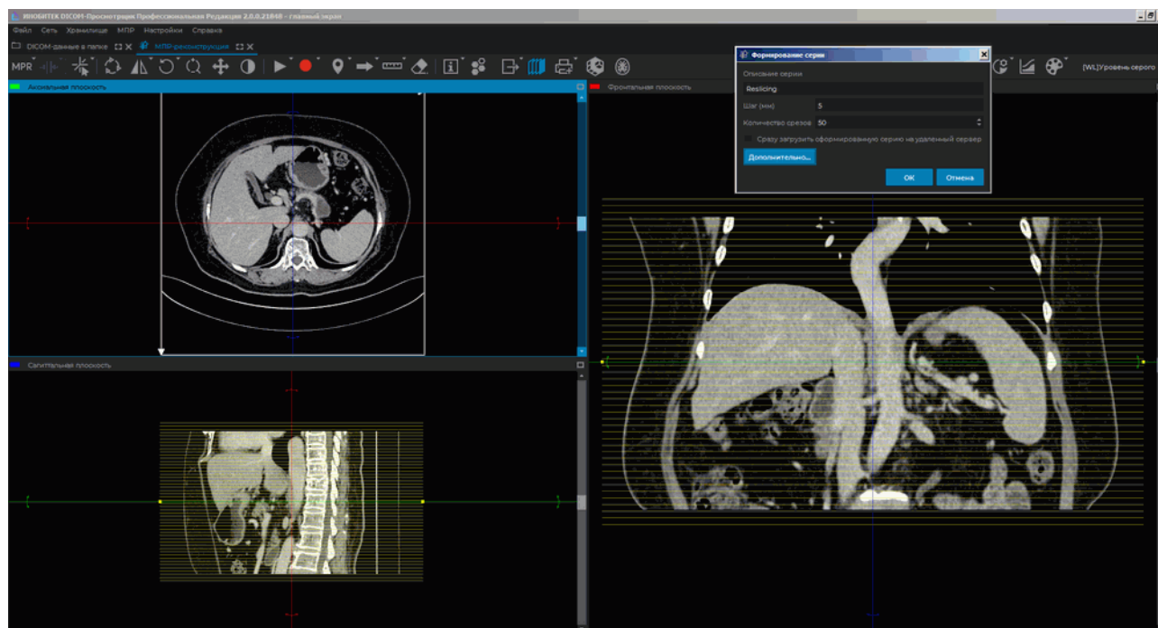
Рис. 5.26: Формирование серии
