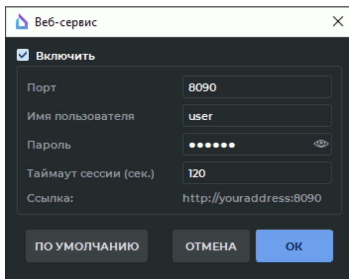
Рис. 13.3: Диалог «Веб-сервис»
