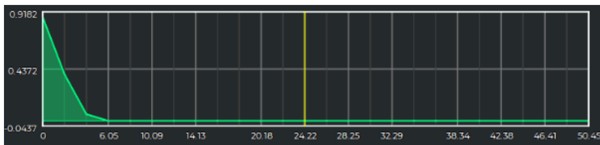
Рис. 2.43: Коэффициент осцилляций 0,01
