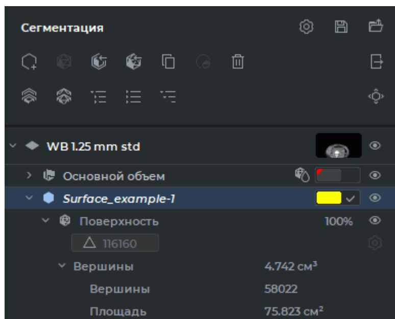
Рис. 6.17: Импортированная поверхность
