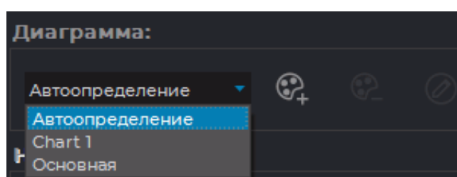
Рис. 2.78: Список диаграмм
