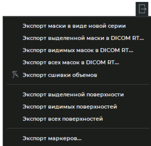
Рис. 4.13: Меню экспорта
