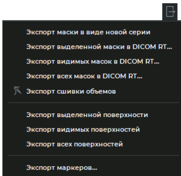
Рис. 6.18: Меню экспорта
