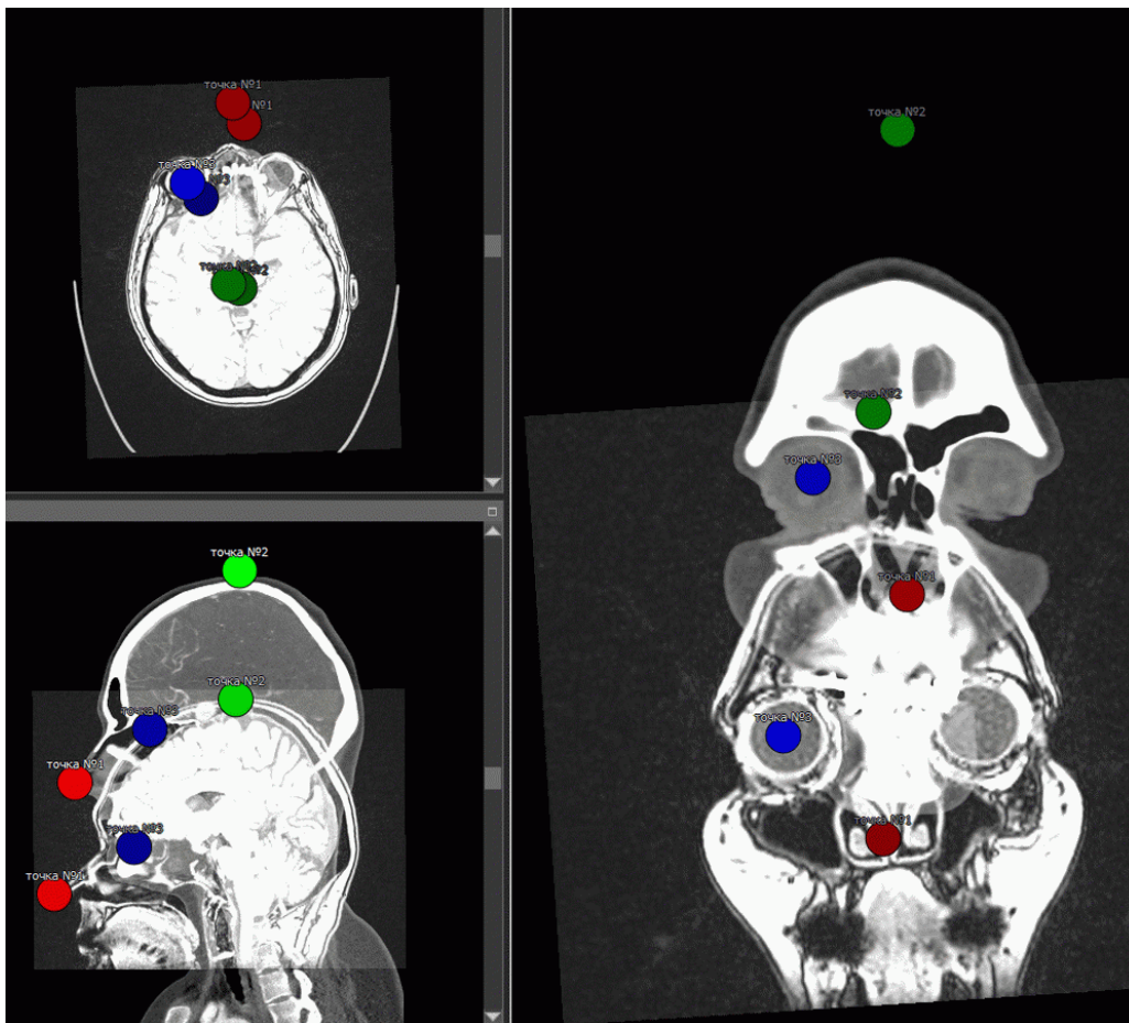
Рис. 4.6: Опорные точки
