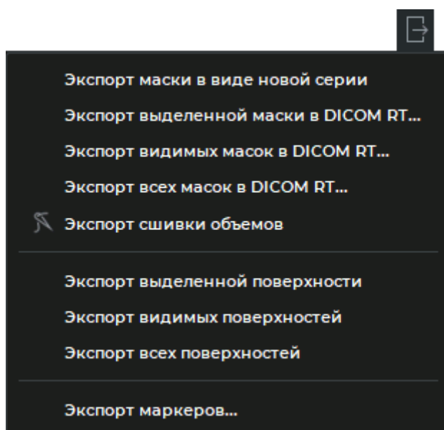
Рис. 6.15: Меню экспорта
