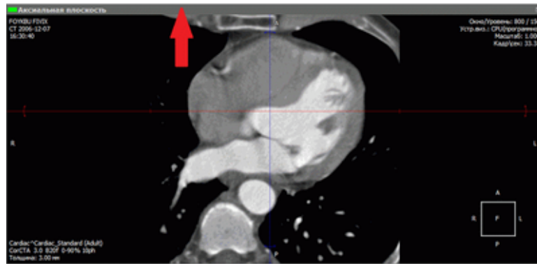
Рис. 5.25: Заголовок окна
