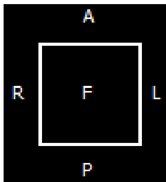
Рис. 2.91: Куб ориентации
