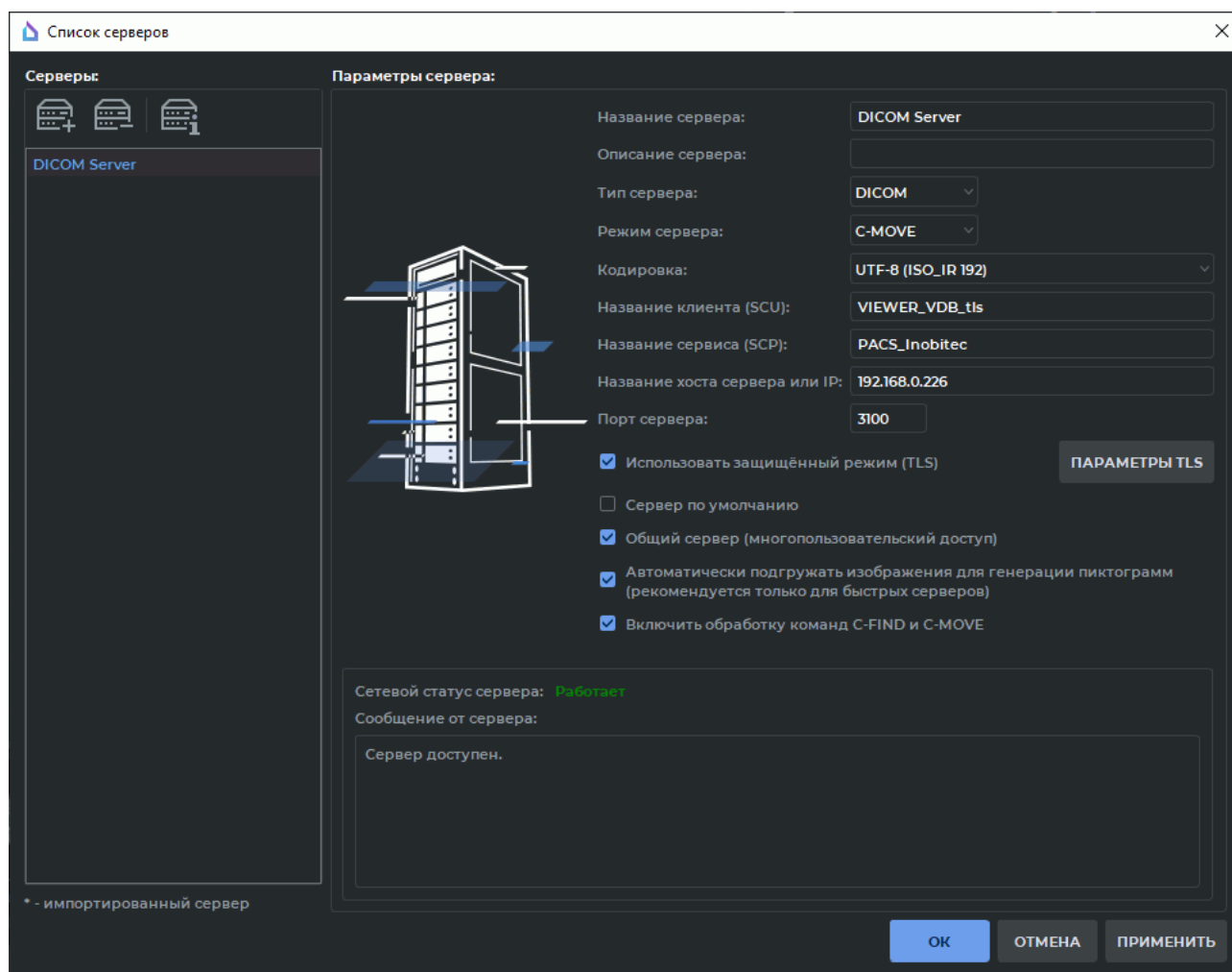
Рис. 13.7: Диалоговое окно настройки соединения с PACS-серверами
