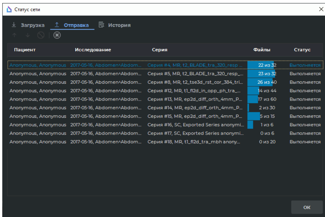
Рис. 13.11: Очередь отправляемых на PACS-сервер исследований
