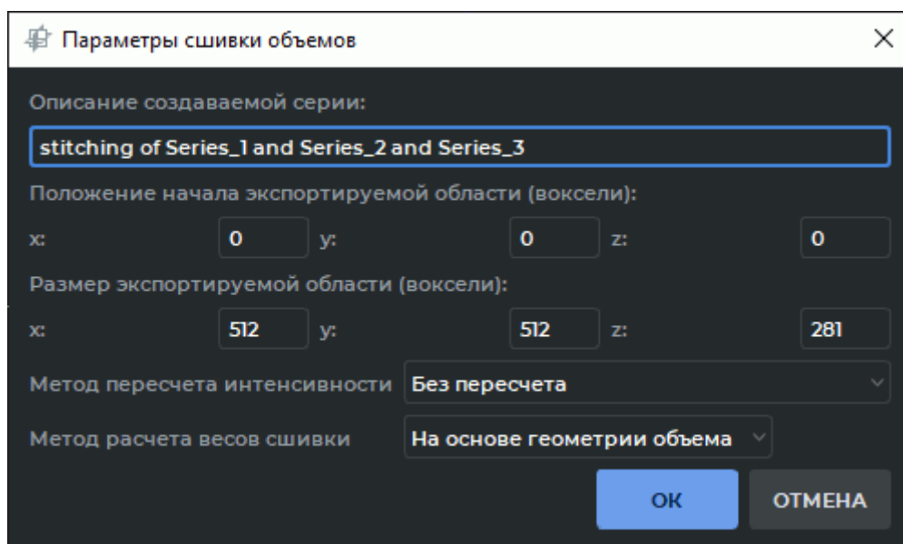
Рис. 4.14: Диалог настройки параметров «сшивки» объёмов
